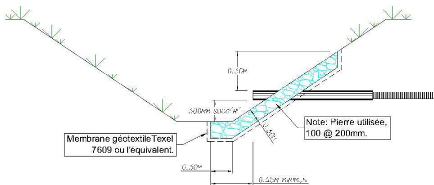
Coupe transversale
